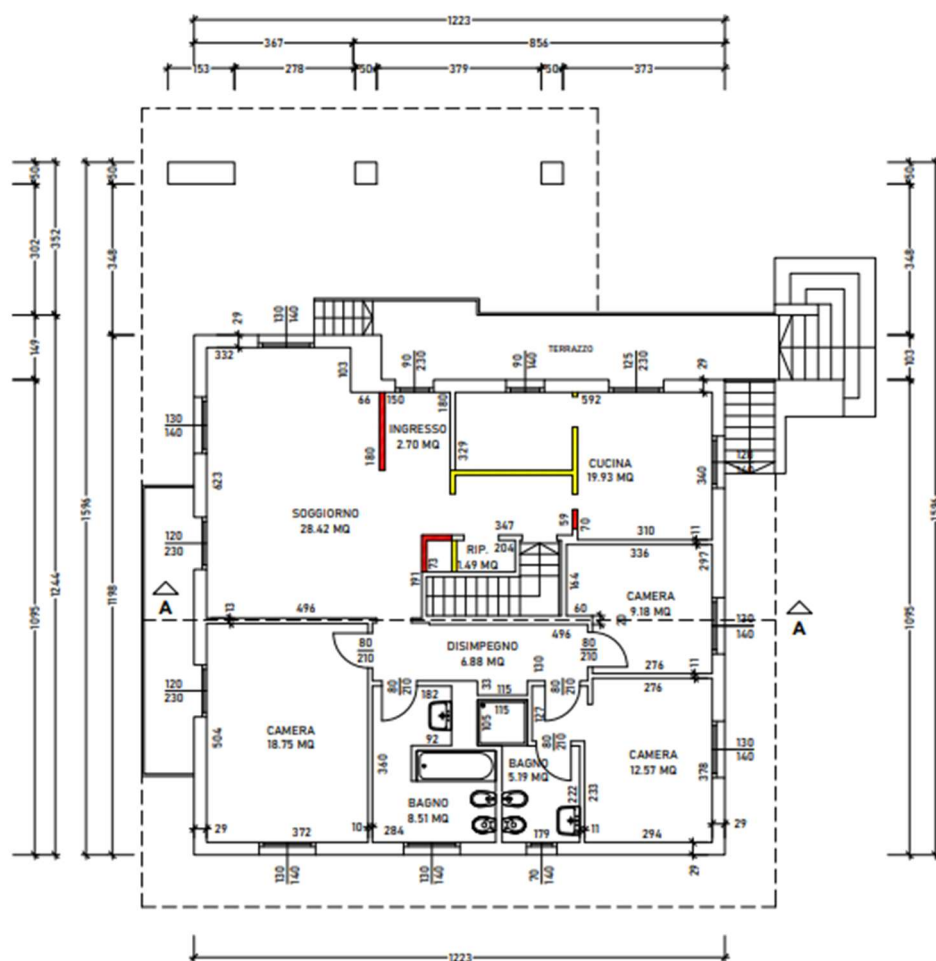
PIANTA PIANO RIALZATO 1/100
